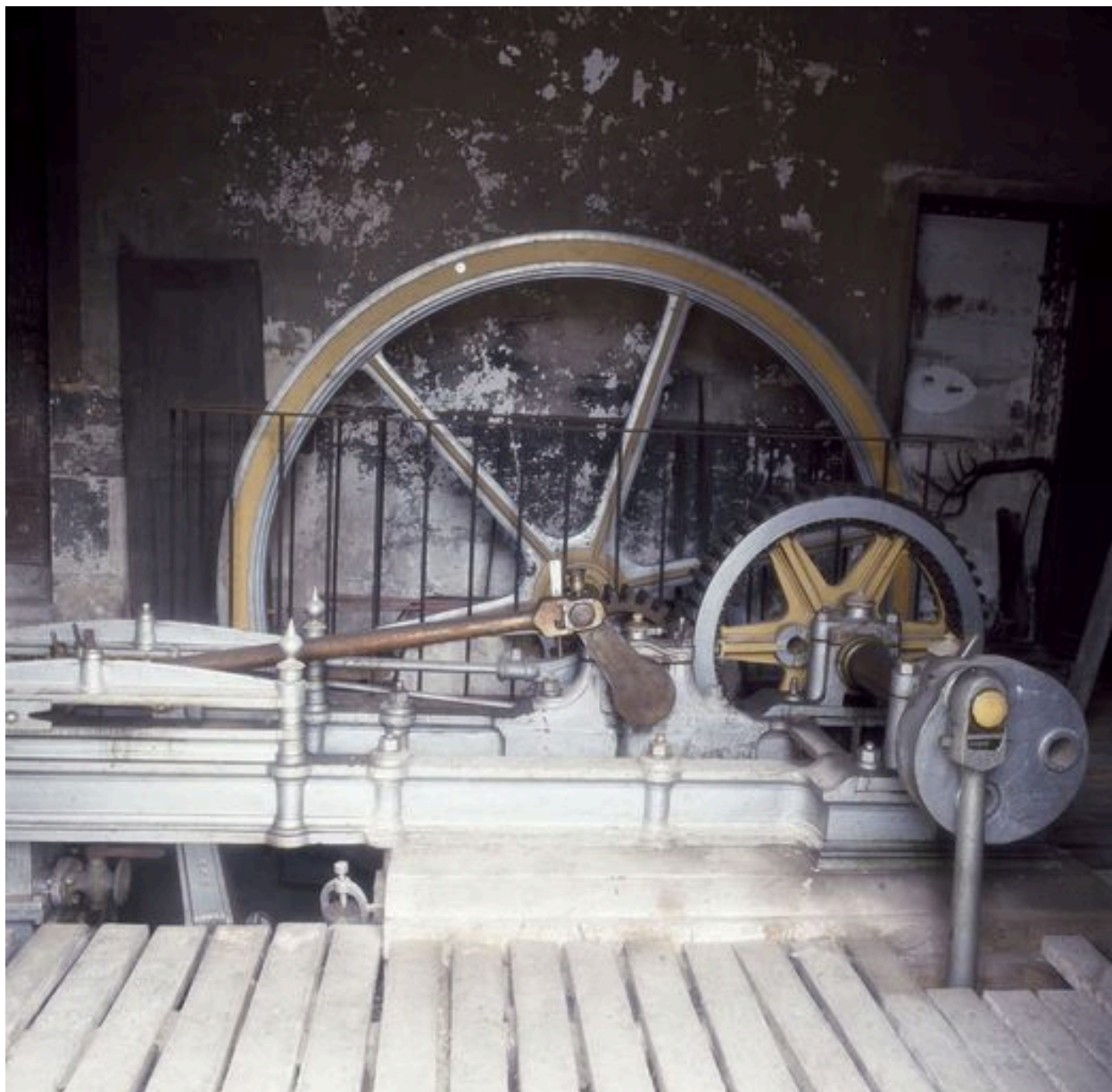
Vue de face du mécanisme : volant, pignon, roue de réducteur, manivelle et bielles du piston.
