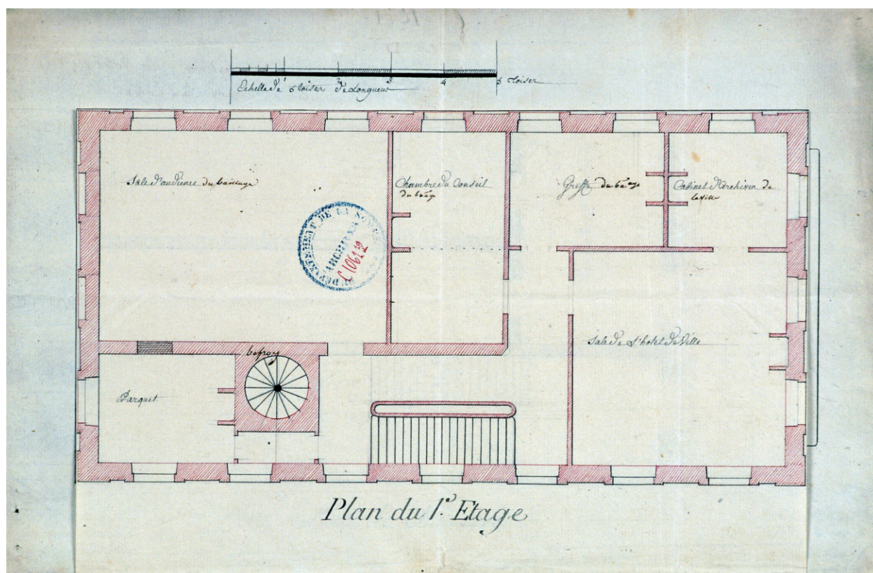
Projet de reconstruction de l'hôtel de ville et de l'auditoire du bailliage royal : plan de distribution du premier étage, 1770 (AD Somme ; 1C_CP_1062/39).
