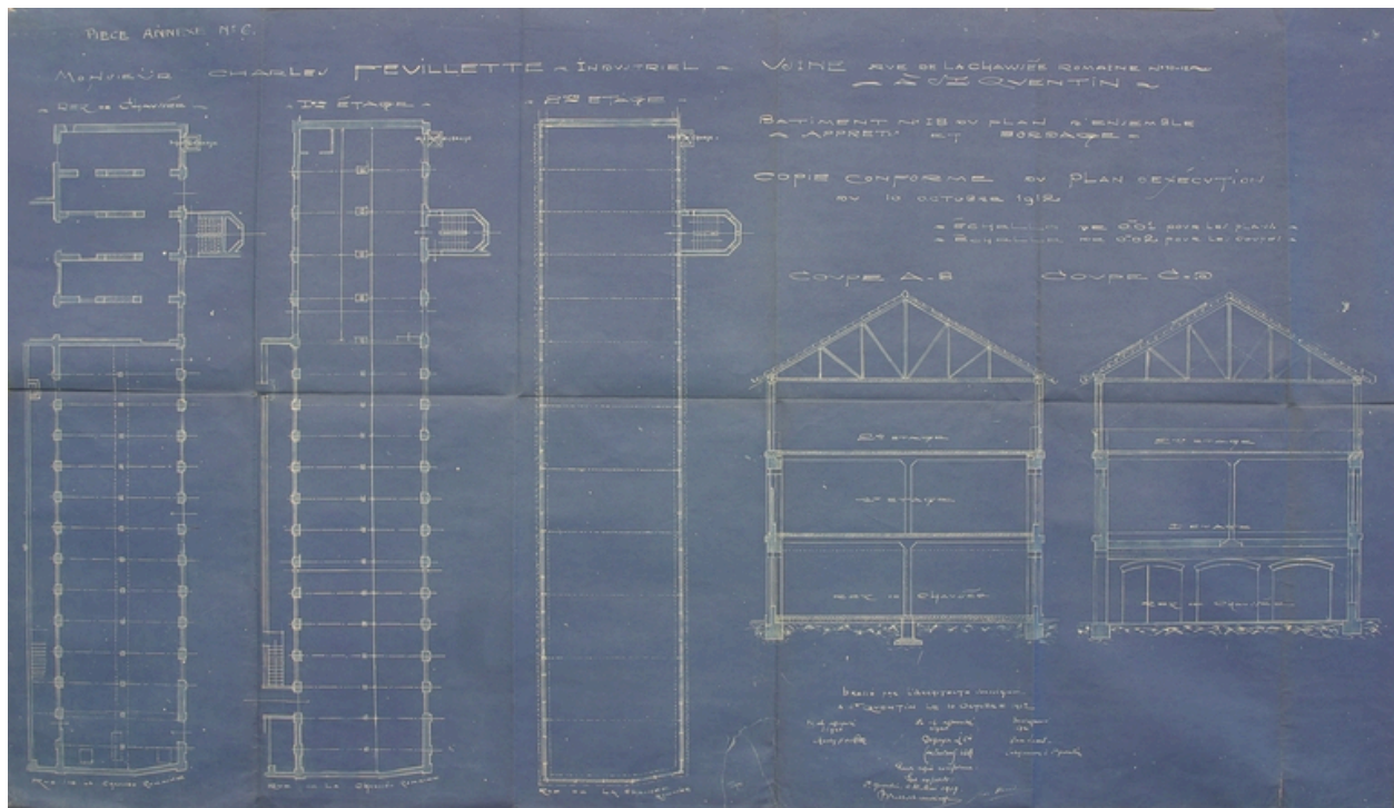
Plan de l'atelier d'apprêt et bordage construit en 1912, restauré en 1919, par Degryse & Cie, Van[hems] (AD Aisne).
