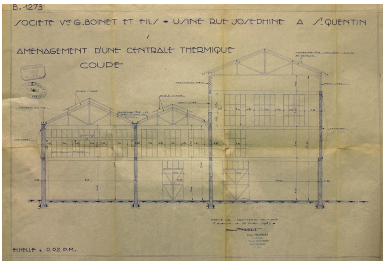
Coupe transversale de la centrale thermique projetée, par Brassart, 1920 (AC Saint-Quentin).
