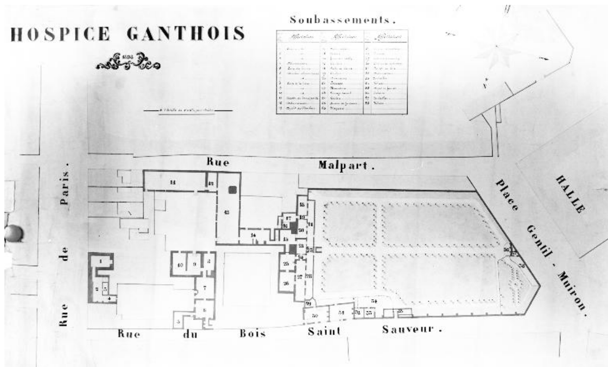
Plan de distribution générale des sous-sols, 1898.
