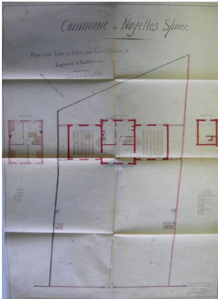
Projet d'école avec école enfantine et logement de l'institutrice en 1882, par Alfred Marchand, plan d'ensemble.
