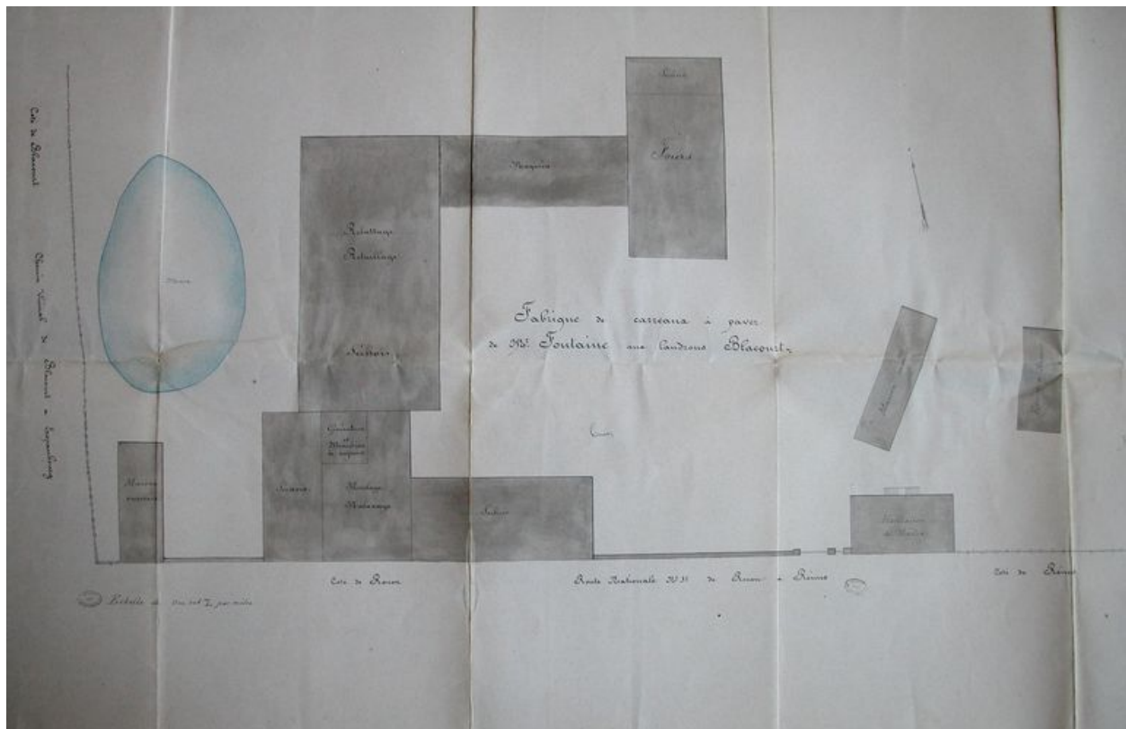
Plan détaillé de la fabrique de carreaux céramiques de M. Fontaine, 1892.
