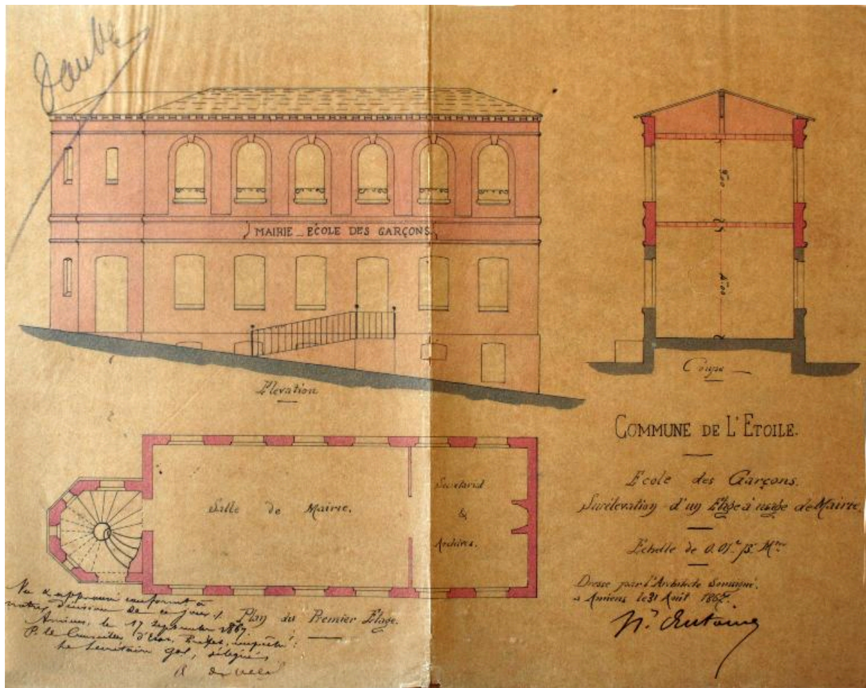
Plan coupe et élévation de l'école des garçons, 1867 (AD Somme ; 99 O 1618).
