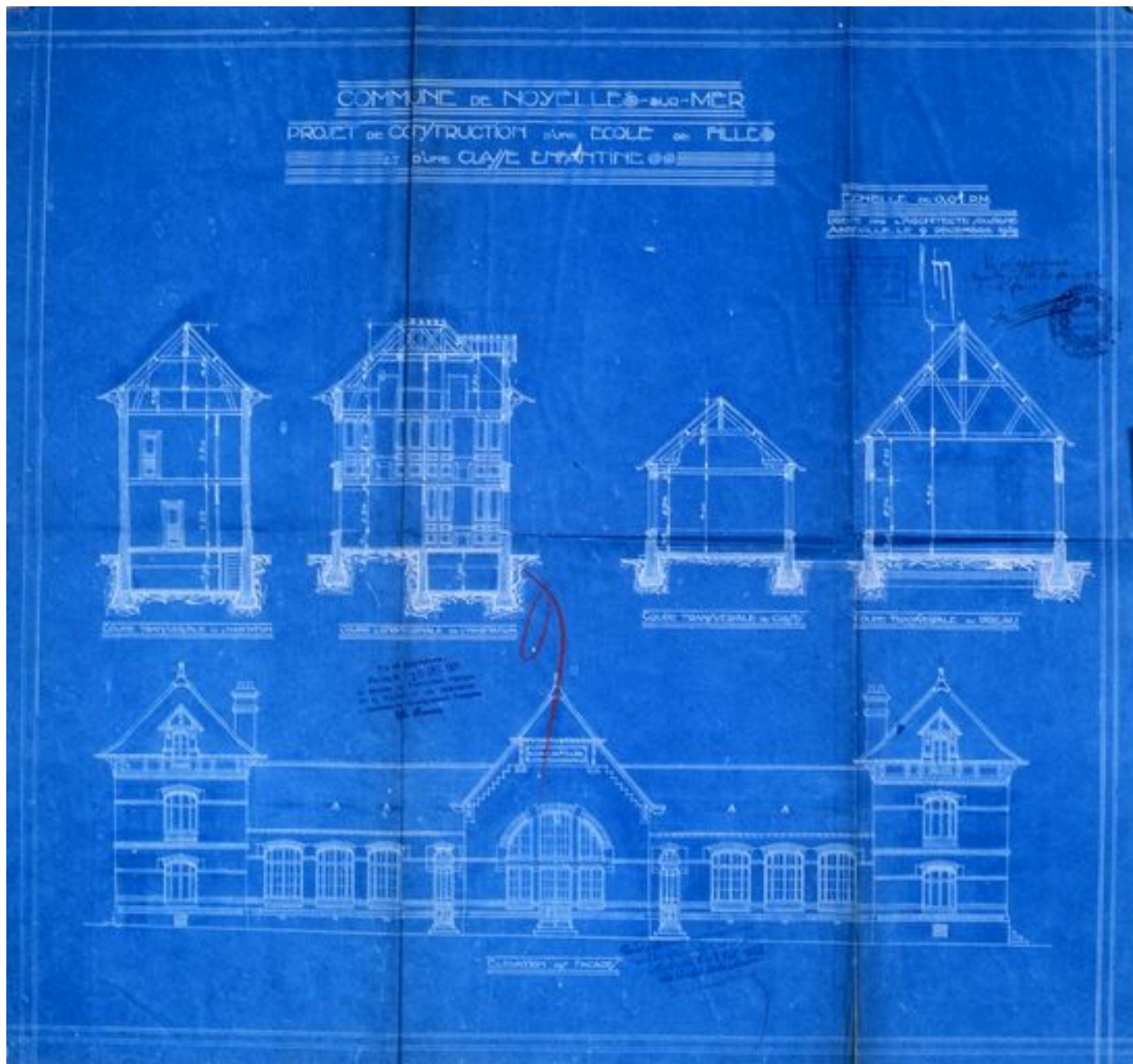
Coupe et élévation de l'école de filles.
