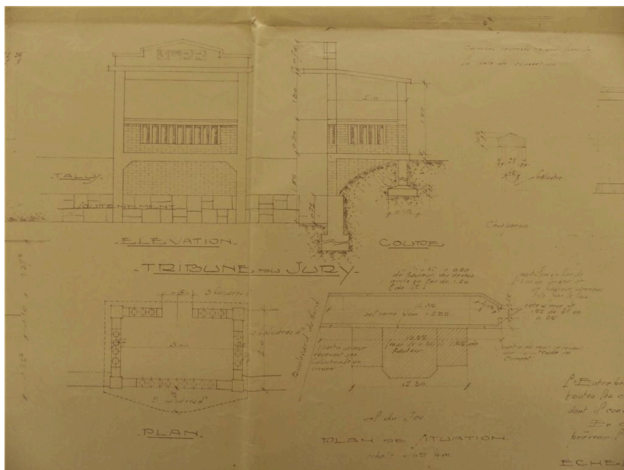
Ville de Roye. Société de Longue paume de Roye. Reconstruction du châlet et de la tribune du jury. Tribune du jury : élévation, coupe et plan. A. Coël architecte, 1927 (AD Somme ; 99O 3297).
