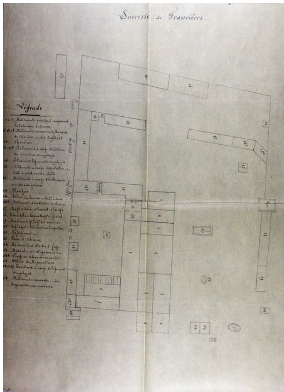
Plan général des bâtiments de la sucrierie avec indication des fonctions de bâtiments, 1893 (AD Oise ; Mp 2474).
