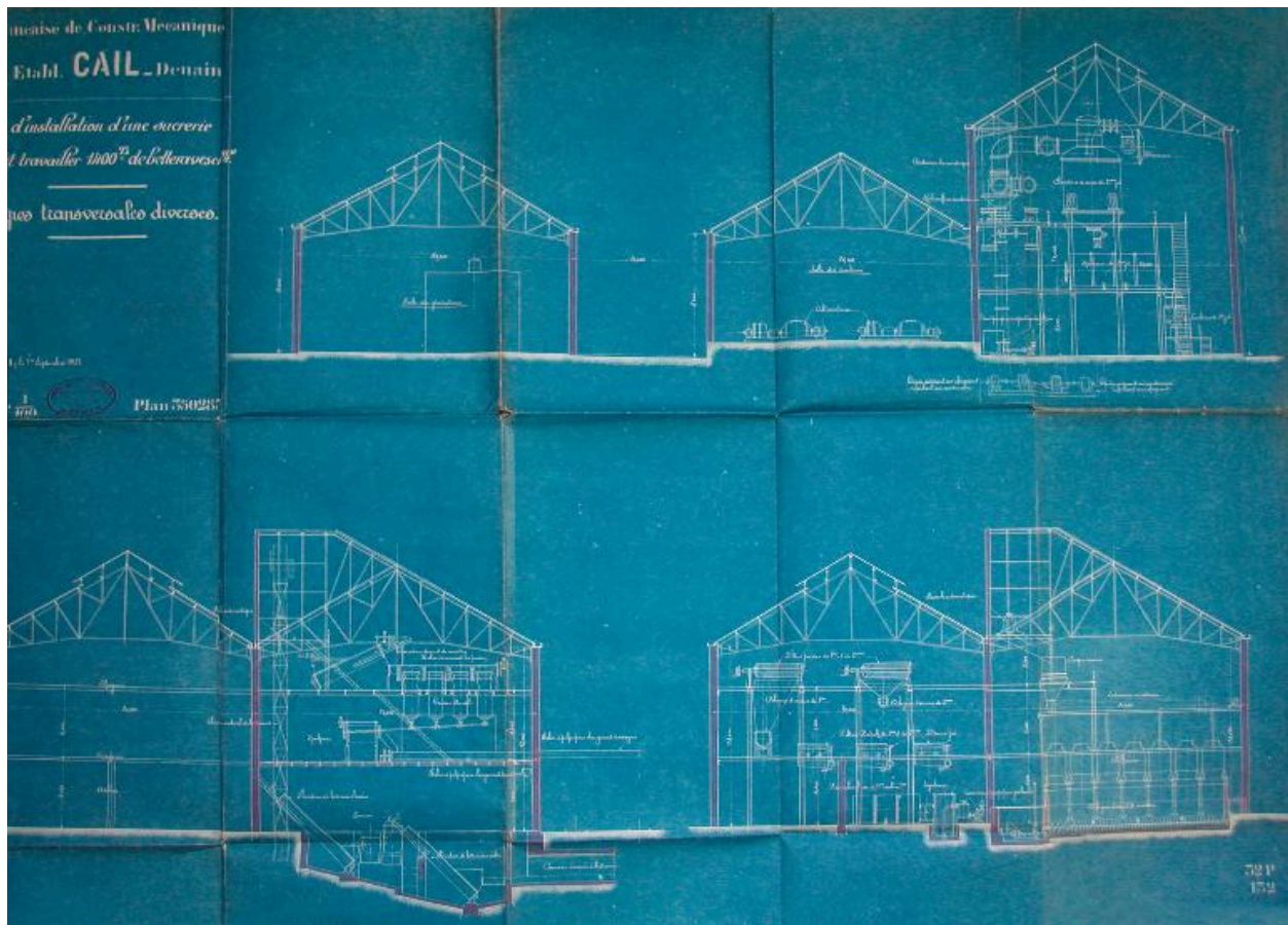
Coupes transversales de la nouvelle sucrierie, 1921 (AD Somme ; 10 R 79).
