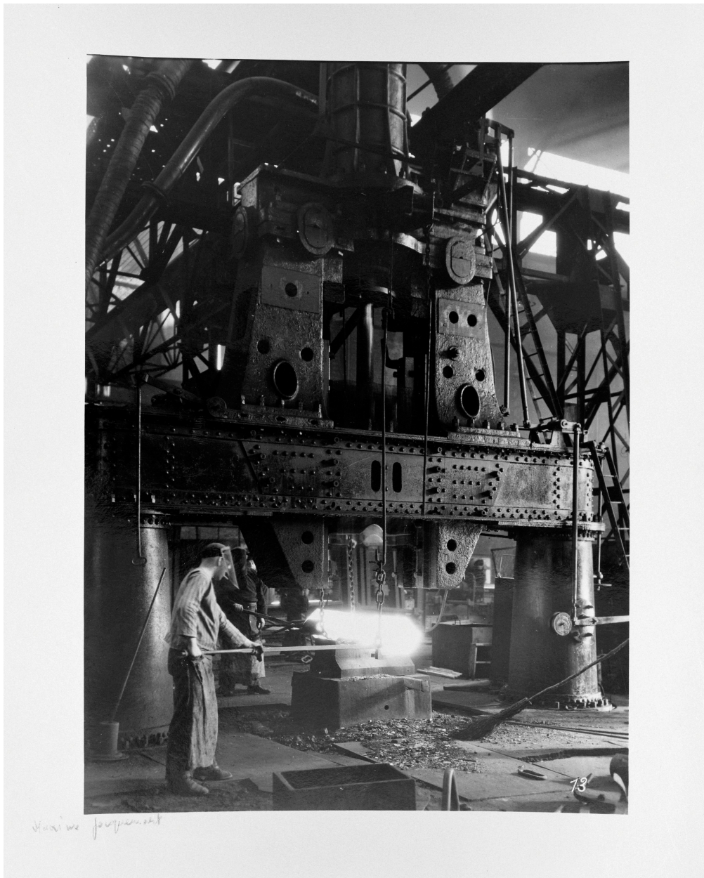
Atelier d'essieux (?) : vue générale d'un marteau-pilon. Photographie ancienne, auteur inconnu sans date (coll. part.).
