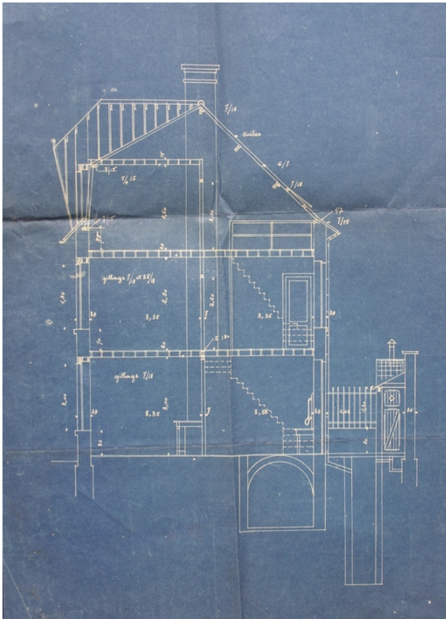
Coupe transversale, 1922.
