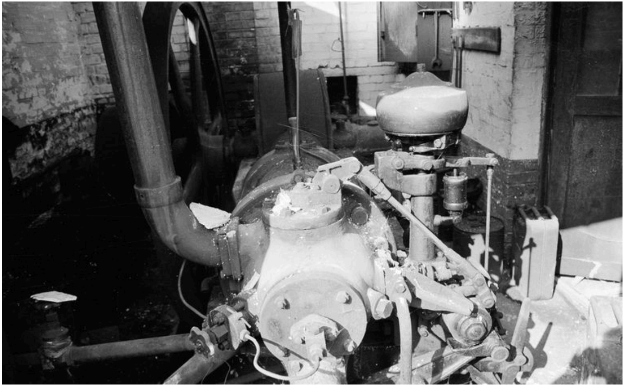
Moteur à pistons à combustion (machine à pression d'huile) : vue partielle de face.
