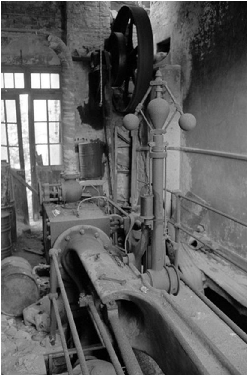
Salle des machines, vue intérieure : machine à vapeur, vers 1990.
