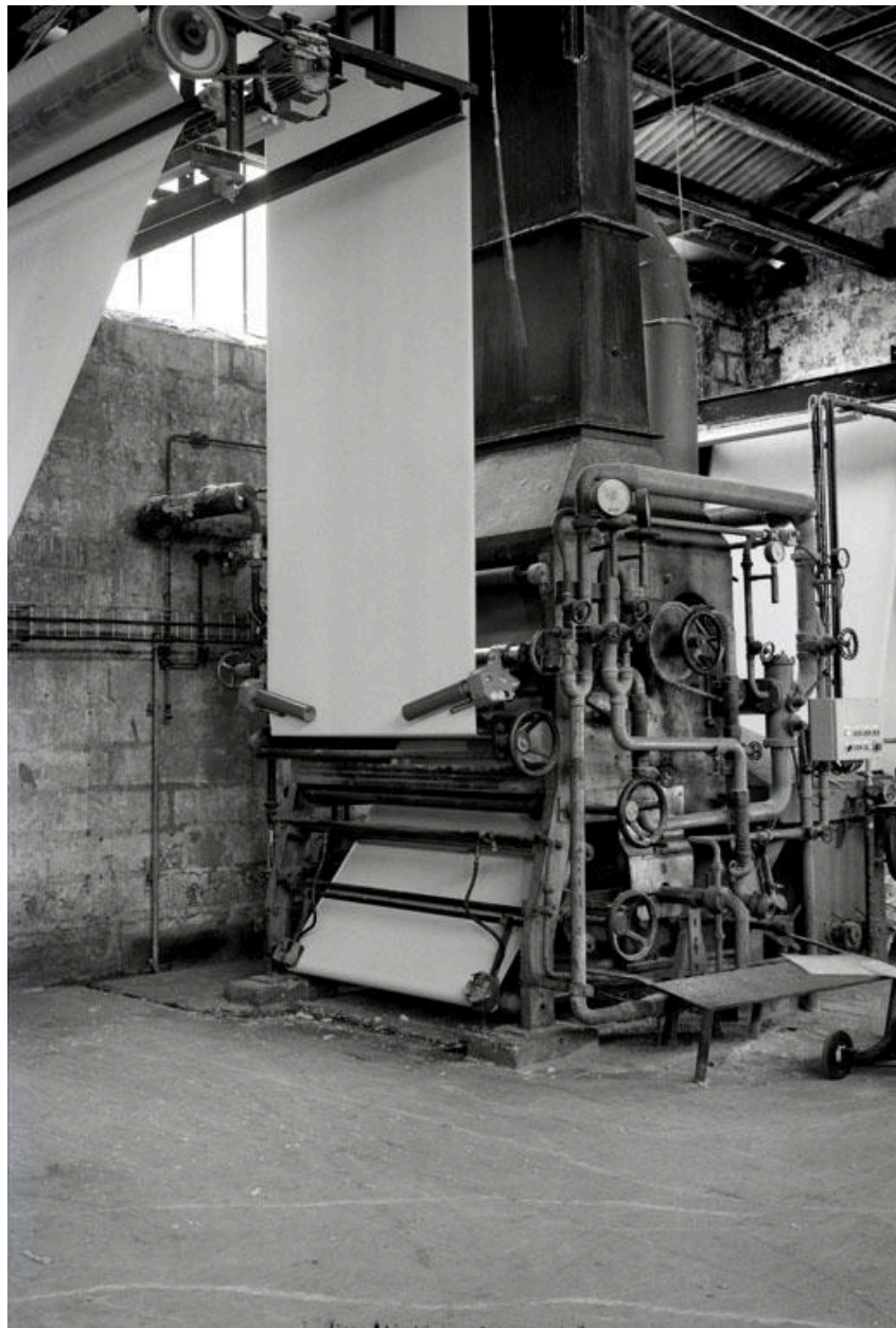
Détail de la machine à griller.
