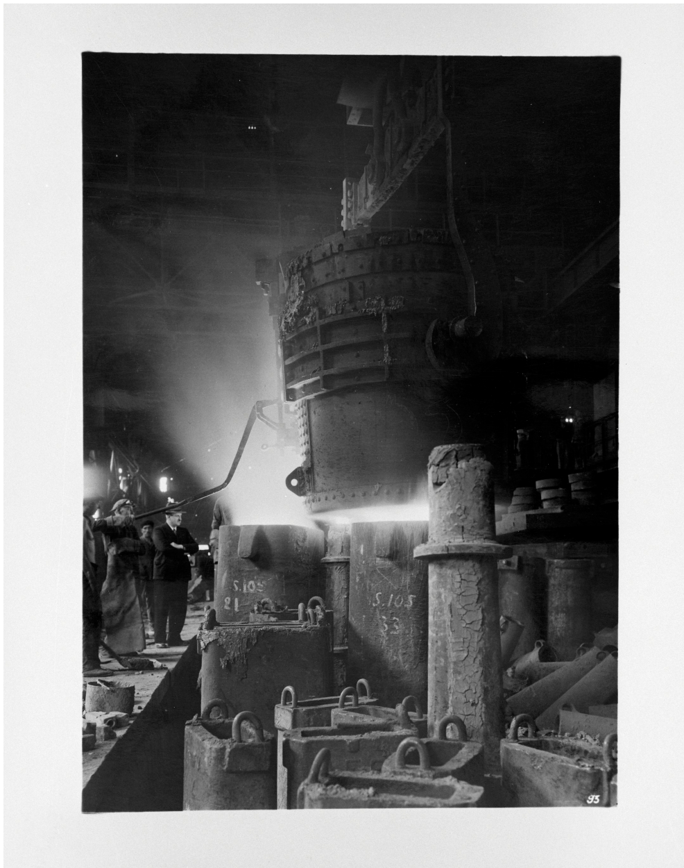
Bassin de coulée de l'aciérie : vue rapprochée de la coulée en lingotières. Photographie ancienne, auteur inconnu, sans date (coll. part.).
