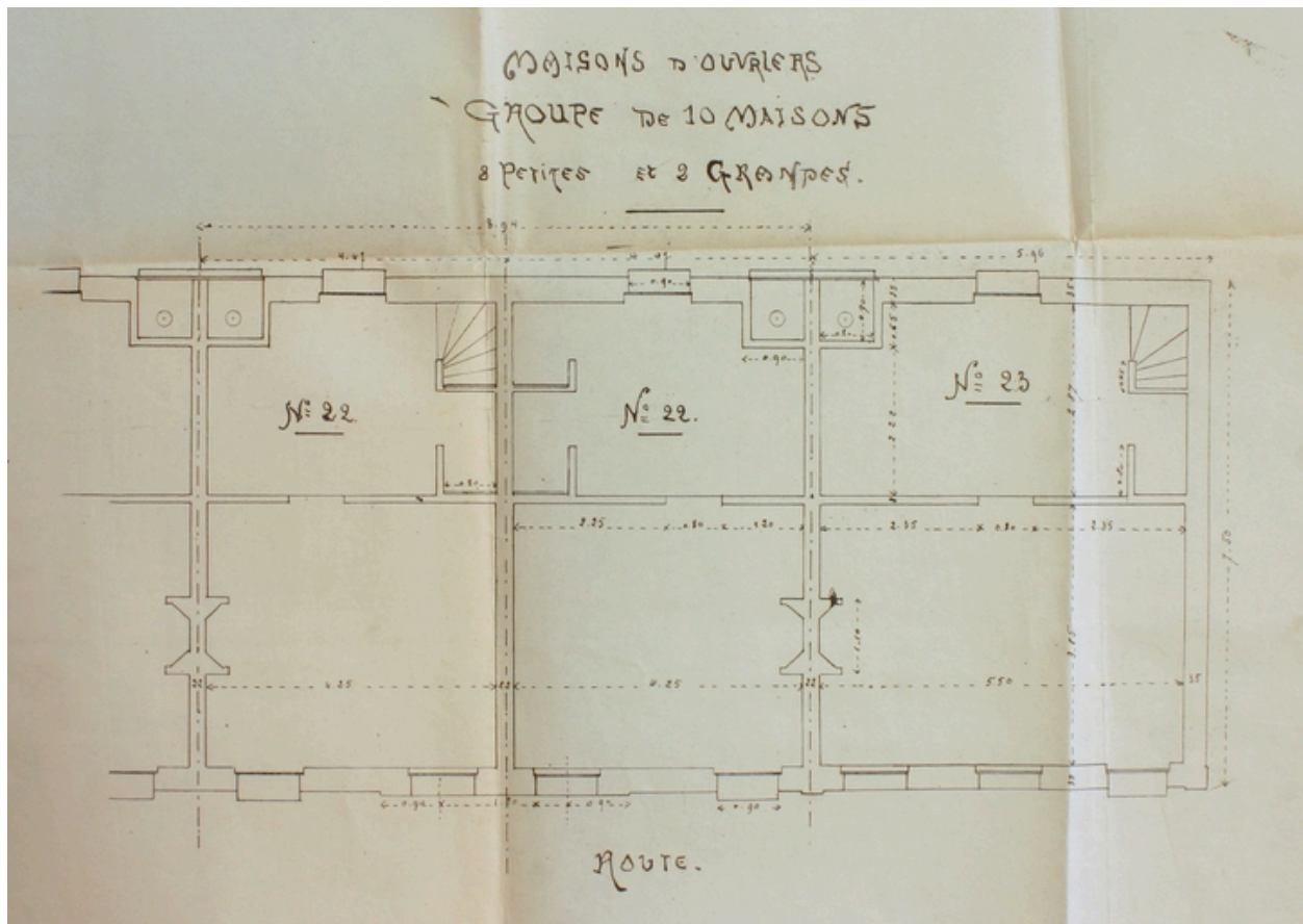
Plan masse des bâtiments de type A (n°22) et de type B (n°23), en 1914 (AD Aisne).
