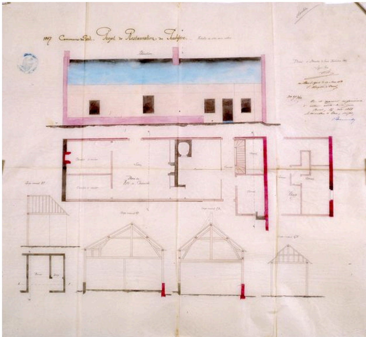
Plan, coupe et élévation dressé par l'entrepreneur Folie en 1867.
