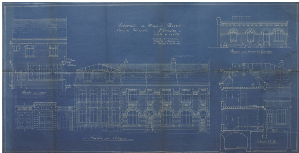
Façades et coupe du logement patronal et des bureaux, par Malgras-Delmas, 1923 (AC Saint-Quentin).
