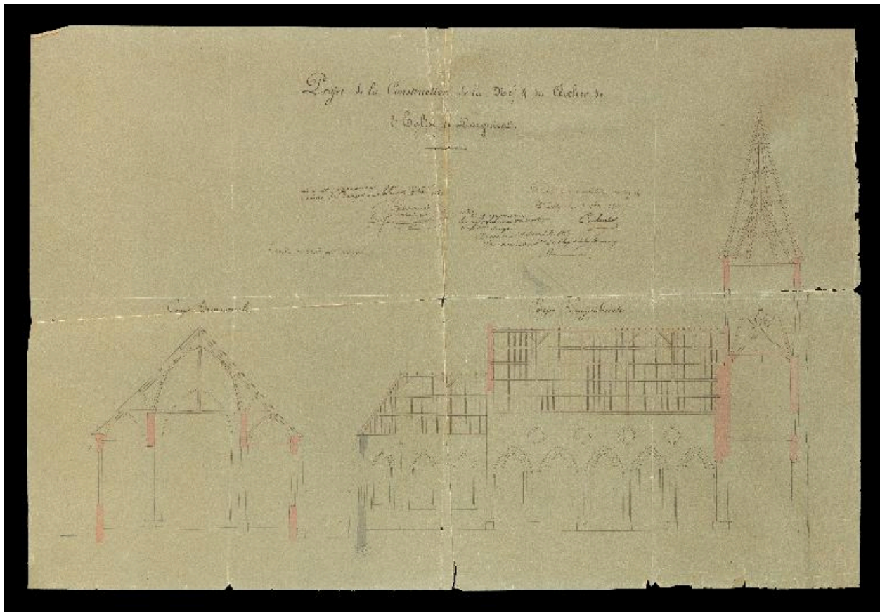
Projet de construction de la nef et du clocher : coupes, par Coulombel, 1859 (AD Somme ; 99 O 1355).
