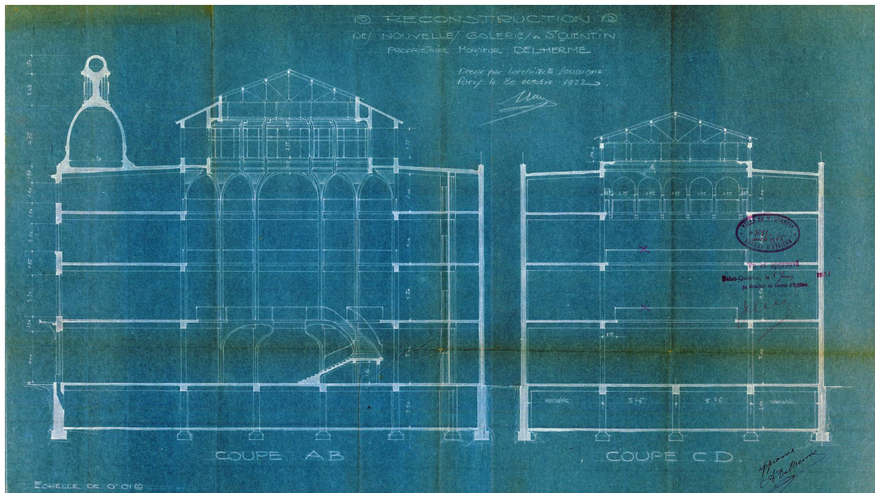
Coupe transversale des deux atriums, octobre 1922 (Archives municipales de Saint-Quentin).
