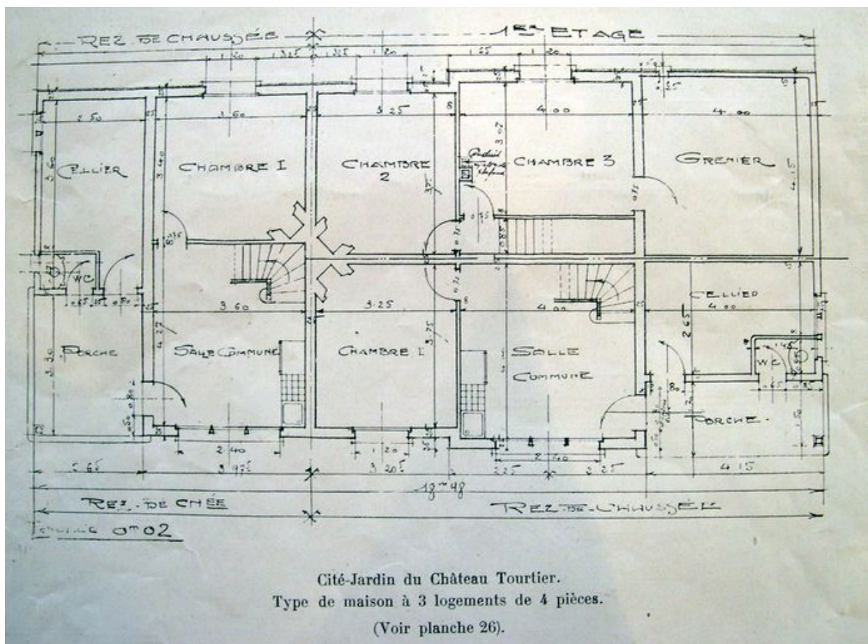
Type de maison à 3 logements de 4 pièces. Plan du rez-de-chaussée et de l'étage (pl. 26) La construction Moderne, n° 4, 24 octobre 1926
