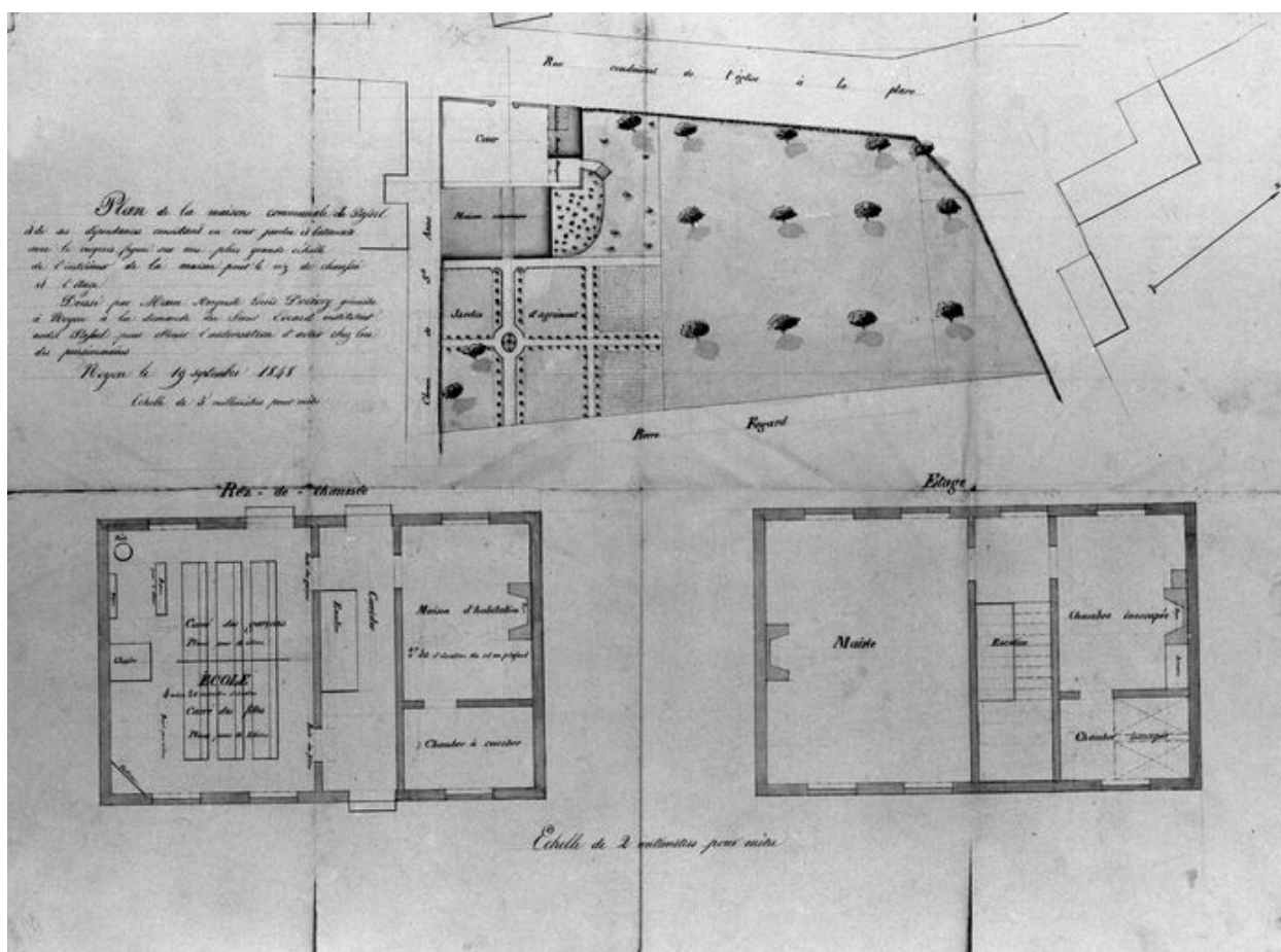
Plan de l'école communale, par L. Derivy, 1848 (AD Oise ; fonds Silvert, 488 021).
