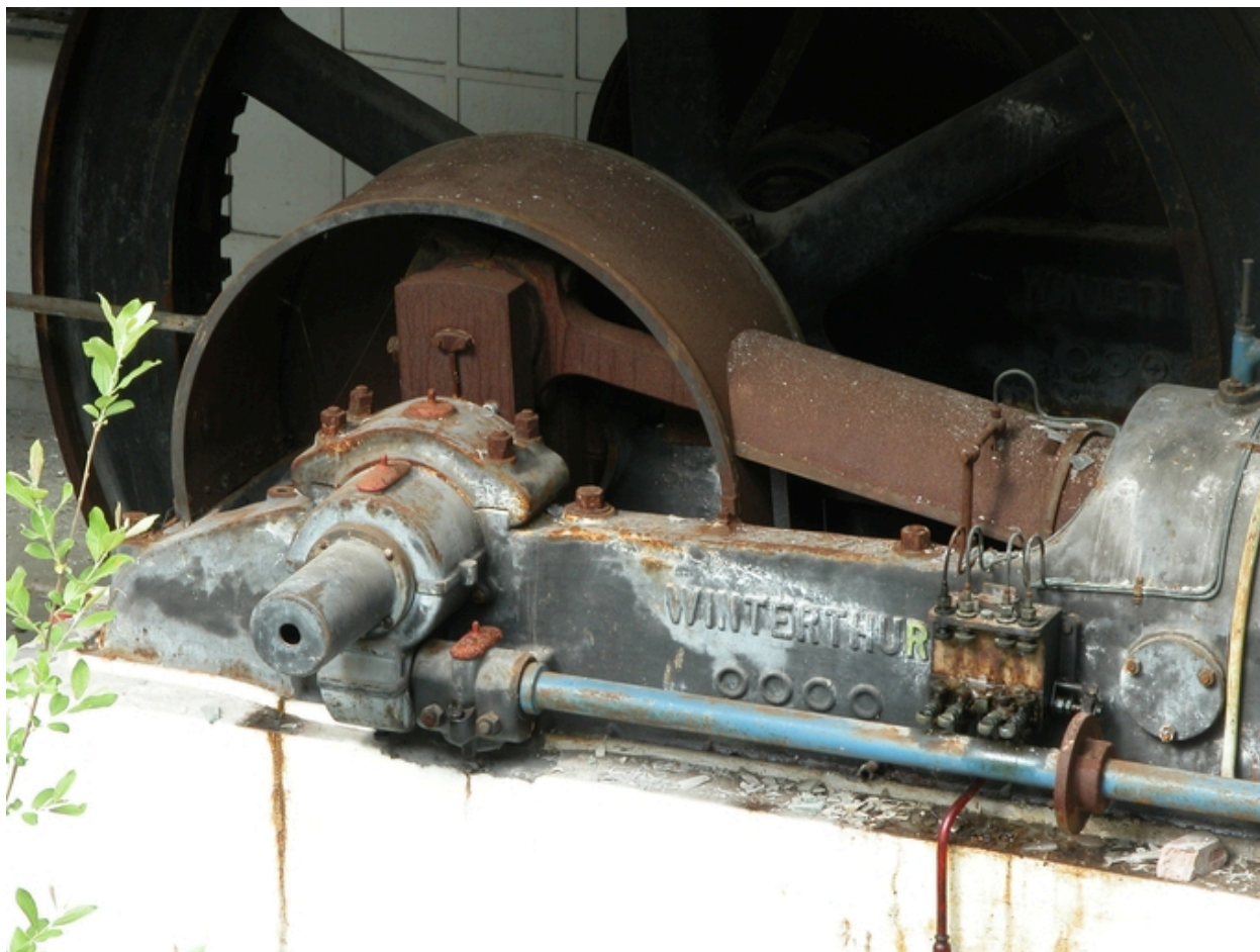
Arbre de transmission, axe du volant, arbre de distribution (peint en bleu) et graisseur de la machine.
