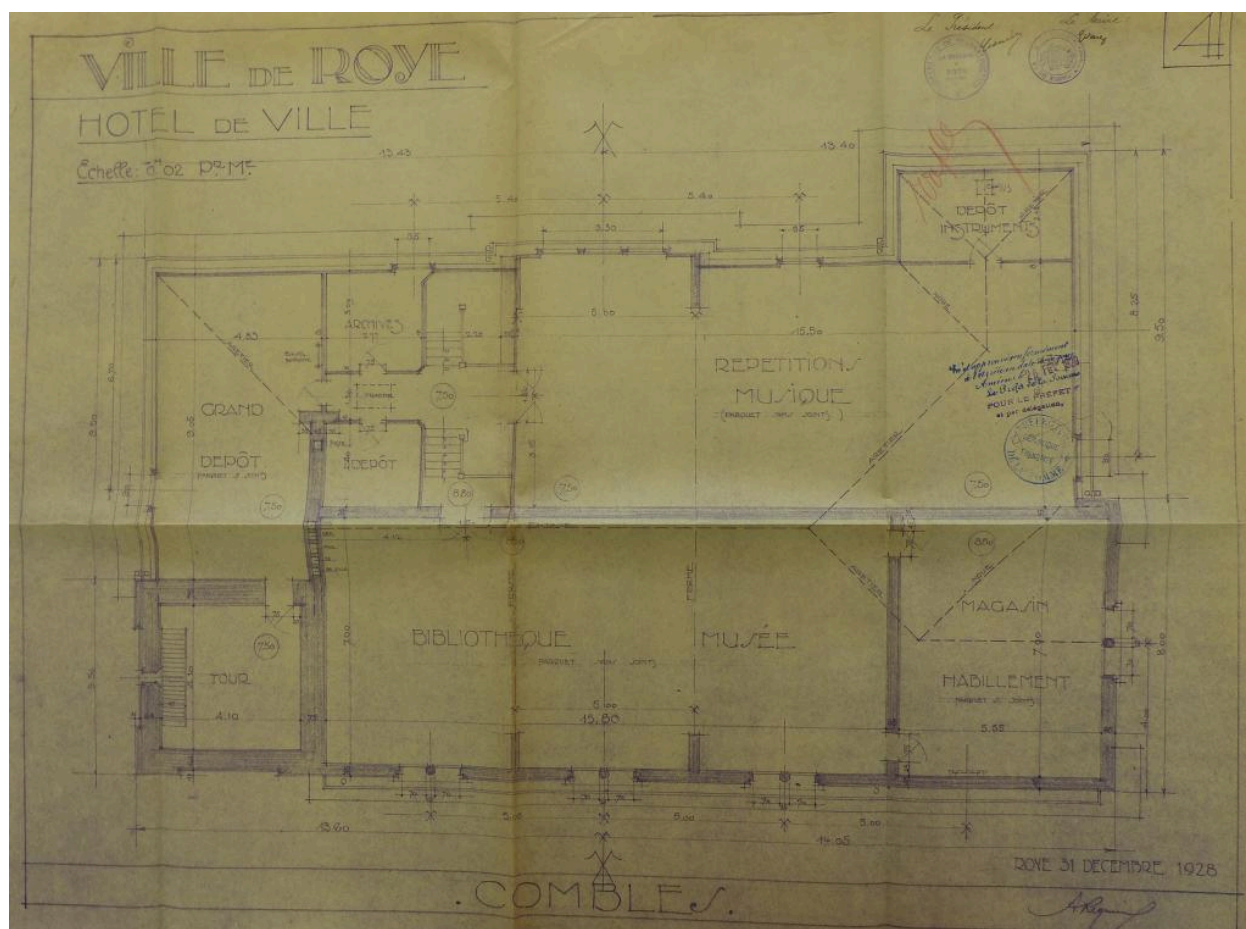
Ville de Roye. Hôtel de ville. Plan des combles. A. Régnier architecte, 1928 (AD Somme ; 99O 3296).
