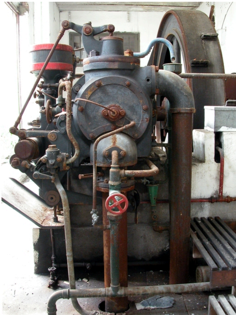
Un moteur de la machine à gaz : systèmes d'admission, d'échappement, etc.
