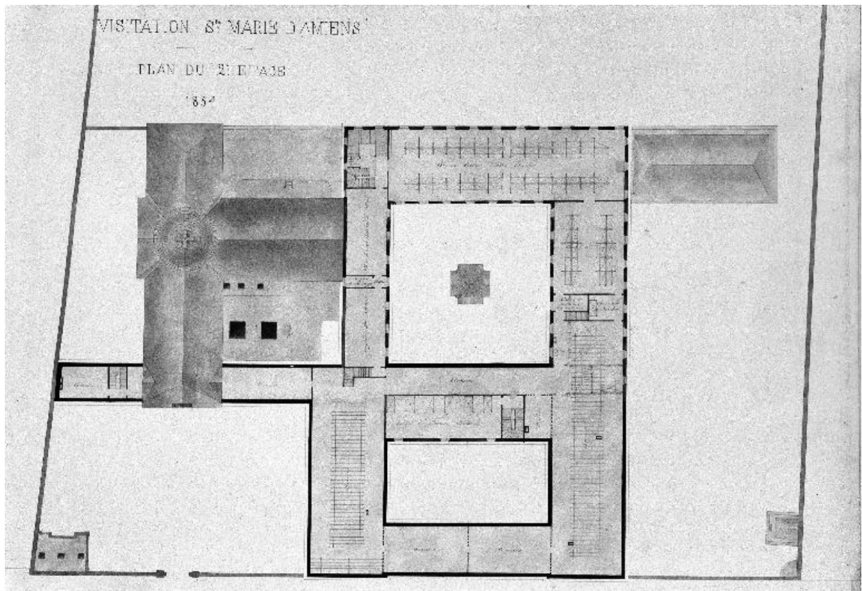
Visitation Sainte-Marie. Plan du 2e étage, par J. Herbault, 1854 (coll. part.).
