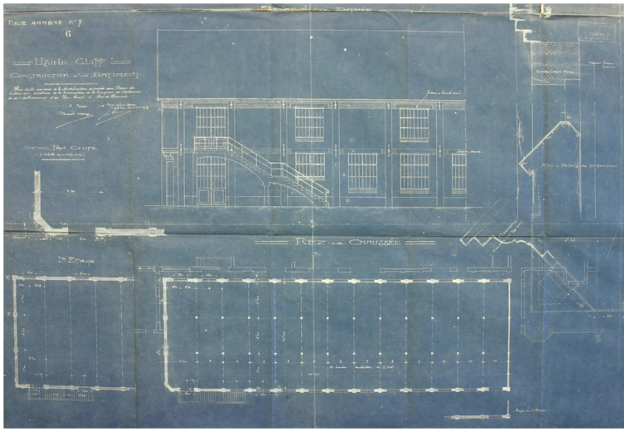
Plan de l'atelier de blanchiment en cours de construction en 1914, par Brassart-Mariage, mai 1919 (AD Aisne).
