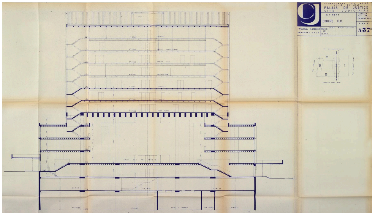
Coupe transversale détaillée en C-C', plan n°A37. 30 avril 1963 (AD Nord : 1348 W 2).
