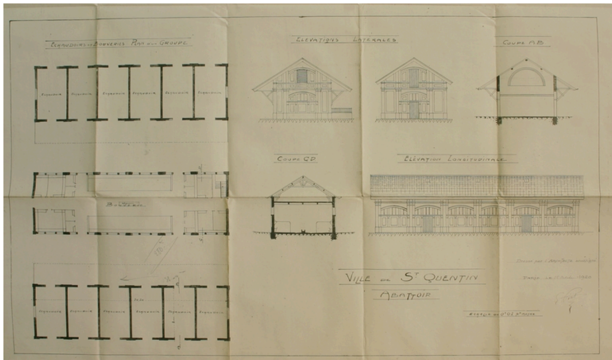
Plans des échaudoirs et des bouvieries construits en 1893, par Piat, 1920 (AD Aisne).
