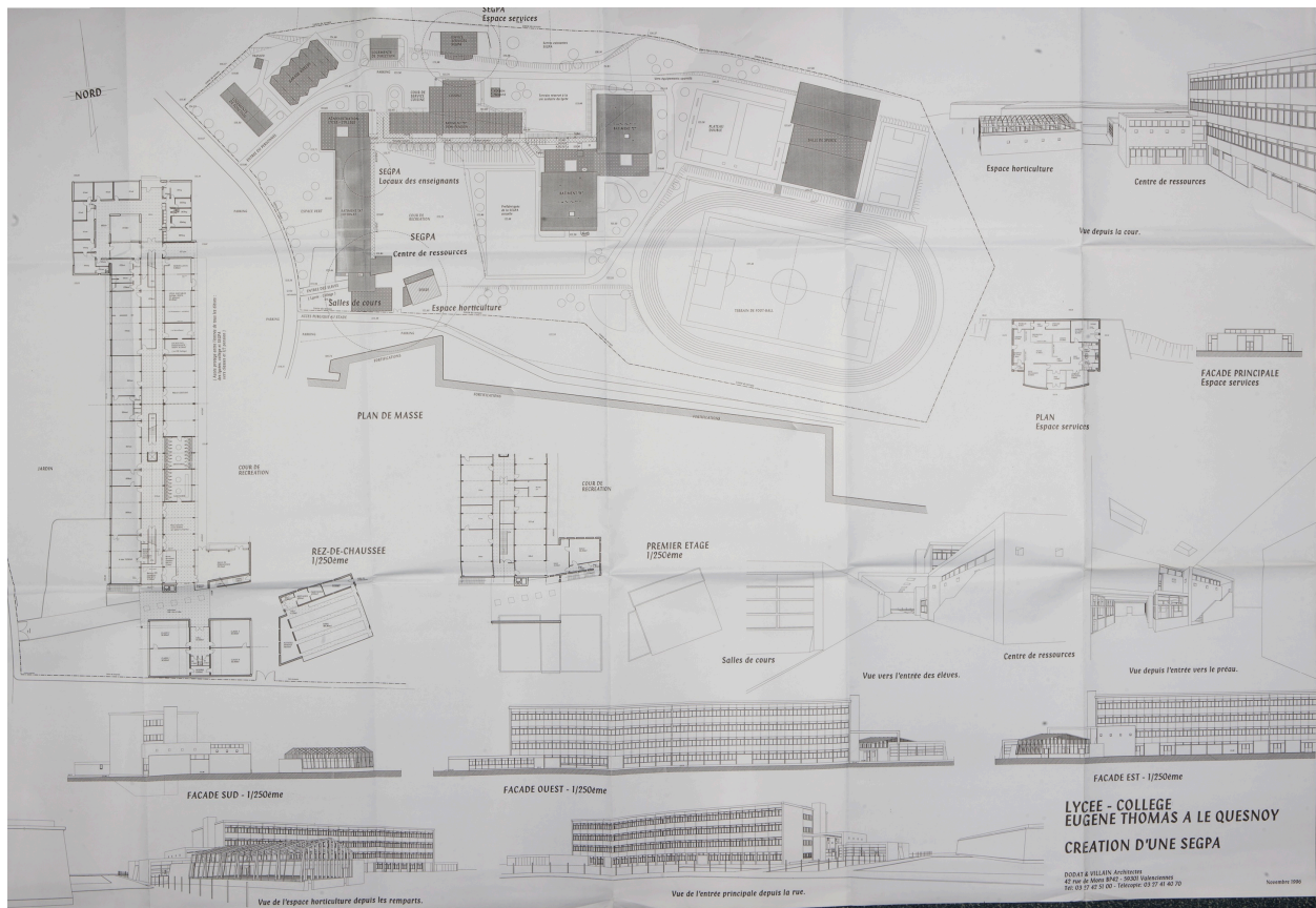
SEGPA : plan masse d'implantation, plans et élévation, 1996. (Collection particulière).
