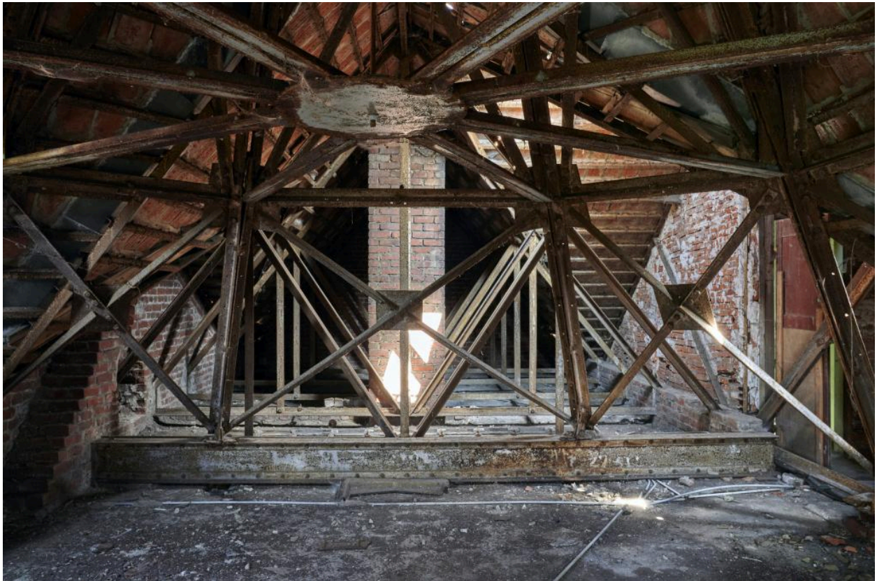
Charpente métallique sous combles du logement du chef d'élevage.
