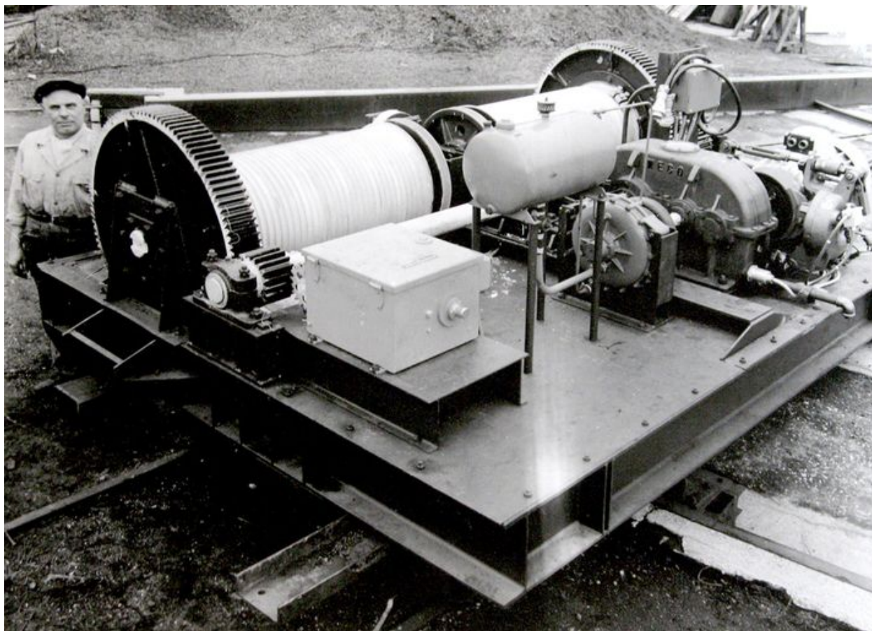
Treuil de manoeuvre et vanne amont pour la centrale EDF de Marckolsheim dans le Bas-Rhin, vers 1950 (AP).
