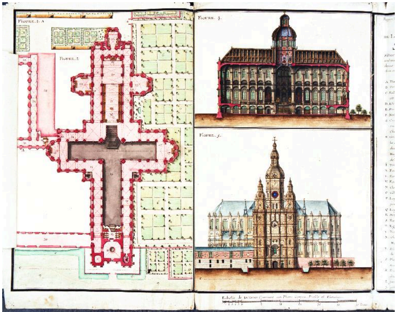
Plan du sous-sol (niveau de la crypte), élévation et coupe de l'église abbatiale de Saint-Amand, Claude Masse, 1725 (Ministère de la Défense, SHD, Vincennes, Fonds du Génie, Atlas Ms 131k, f°84).
