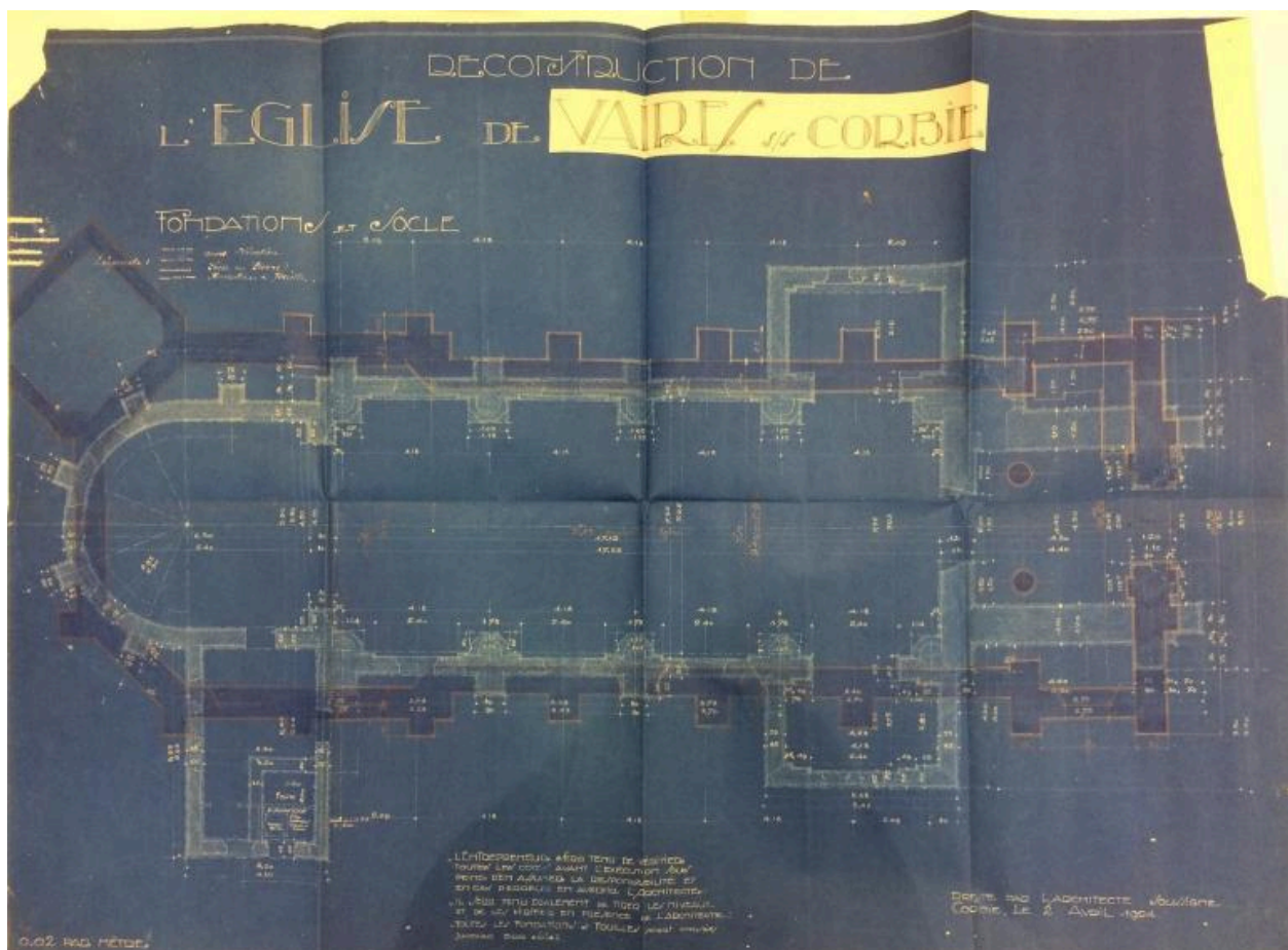
Reconstruction de l'église de Vaire-sous-Corbie. Plan des fondations. 1924 (AD Somme ; 10R 1236).
