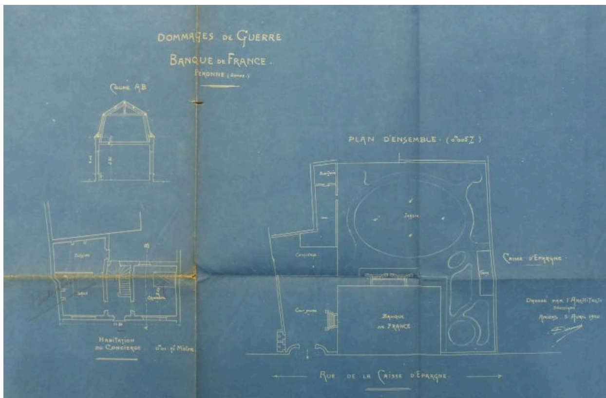
Domage de guerre. Banque de France à Péronne. Plan d'ensemble, plan du logement du concierge et coupe, par Darcourt architecte, 1920 (AD Somme ; 10R 1018).
