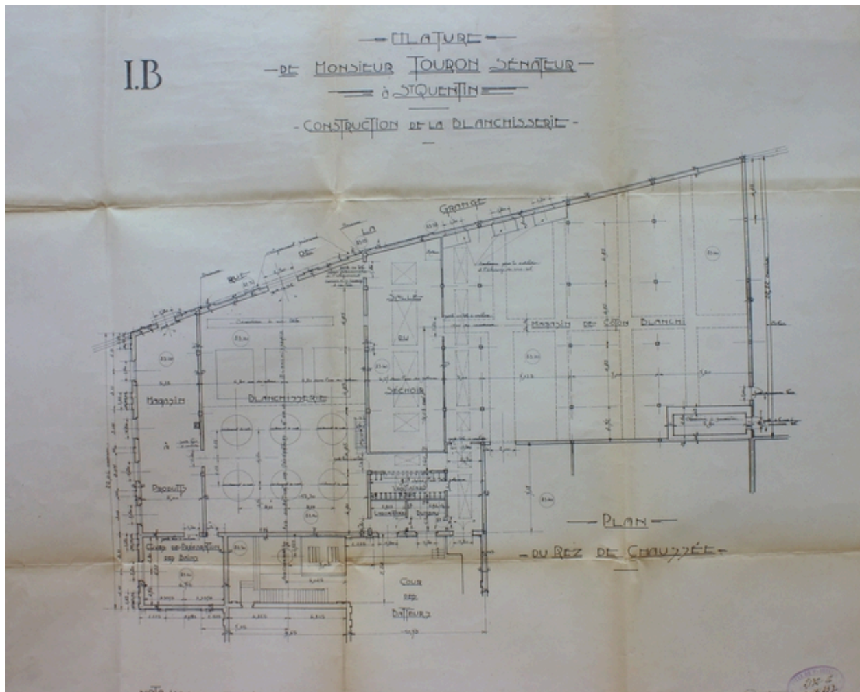
Plan de construction de la blanchisserie, par Narlet (arch.), 1922 (AC Saint-Quentin).
