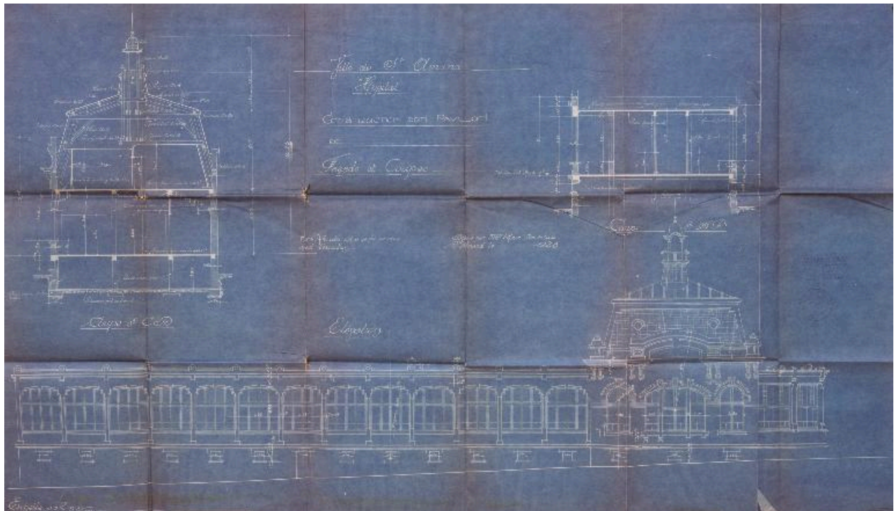
Projet d'un nouveau pavillon, élévation et coupes, Raux architecte 1928 (AH, centre hospitalier de Saint-Amand-les-Eaux).
