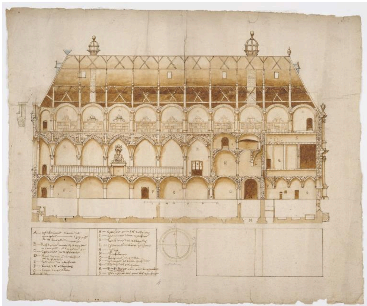
Coupe de l'aile nord du cloître de l'abbaye, vers 1700 (Musée municipal Saint-Amand-les-Eaux).
