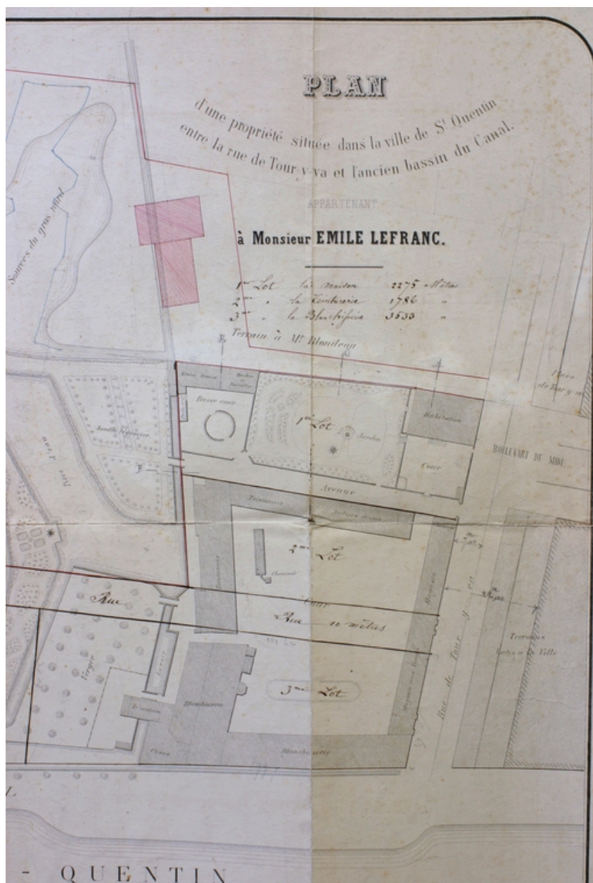
Implantation des bâtiments de l'ancienne usine Lefranc, par Hachet, vers 1870 (AC Saint-Quentin).
