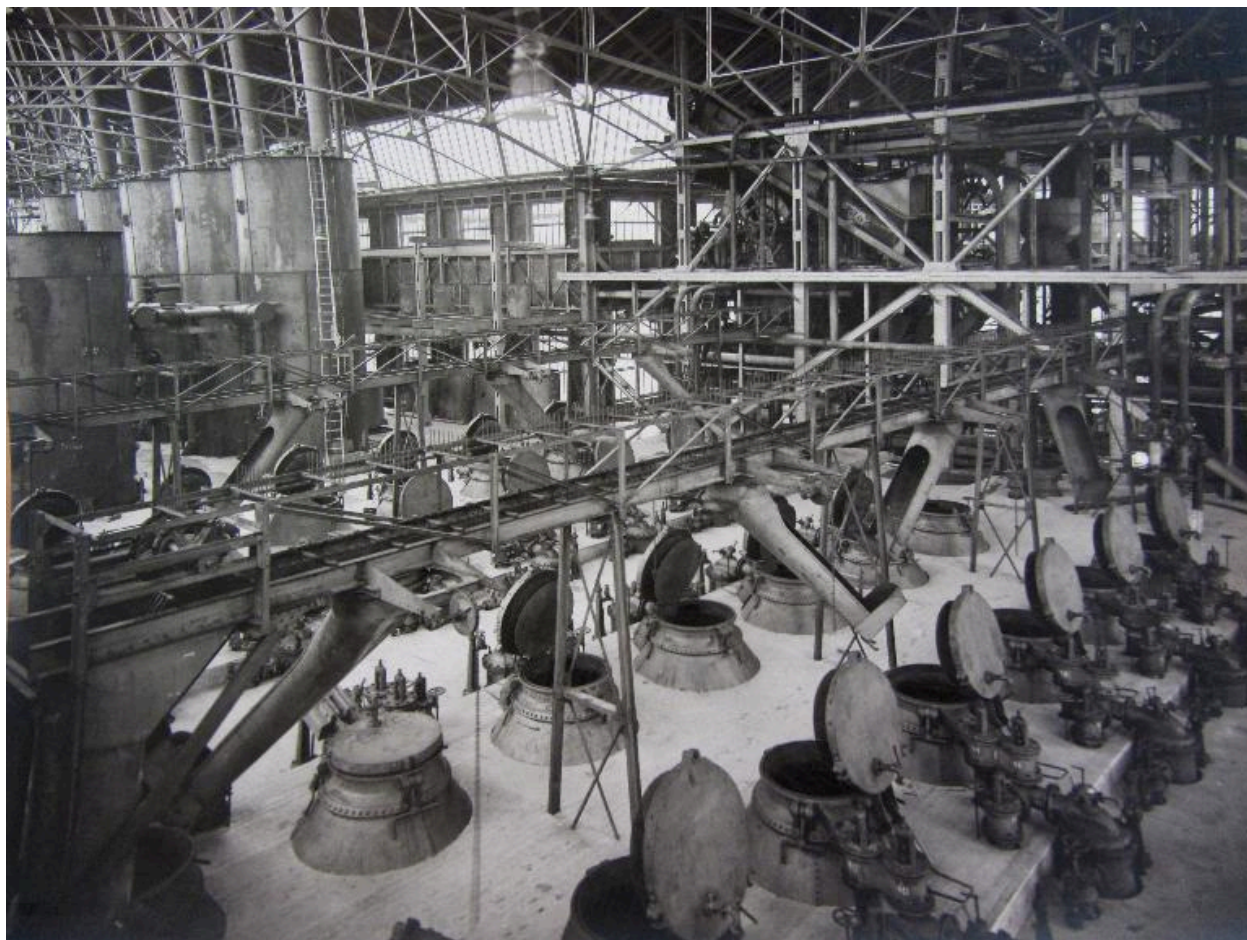
Les vases de diffusion de la sucrierie, 6 novembre 1922 (AD Somme ; 49 Fi 18).
