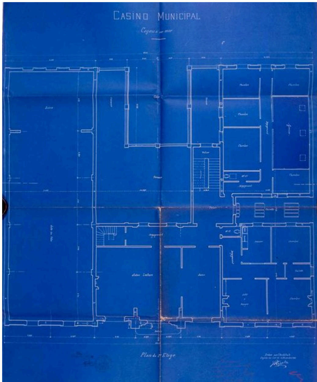
2e casino de Cayeux-sur-Mer, plan du premier étage, par Léon Kämpfer architecte, 1908 (AD Somme).
