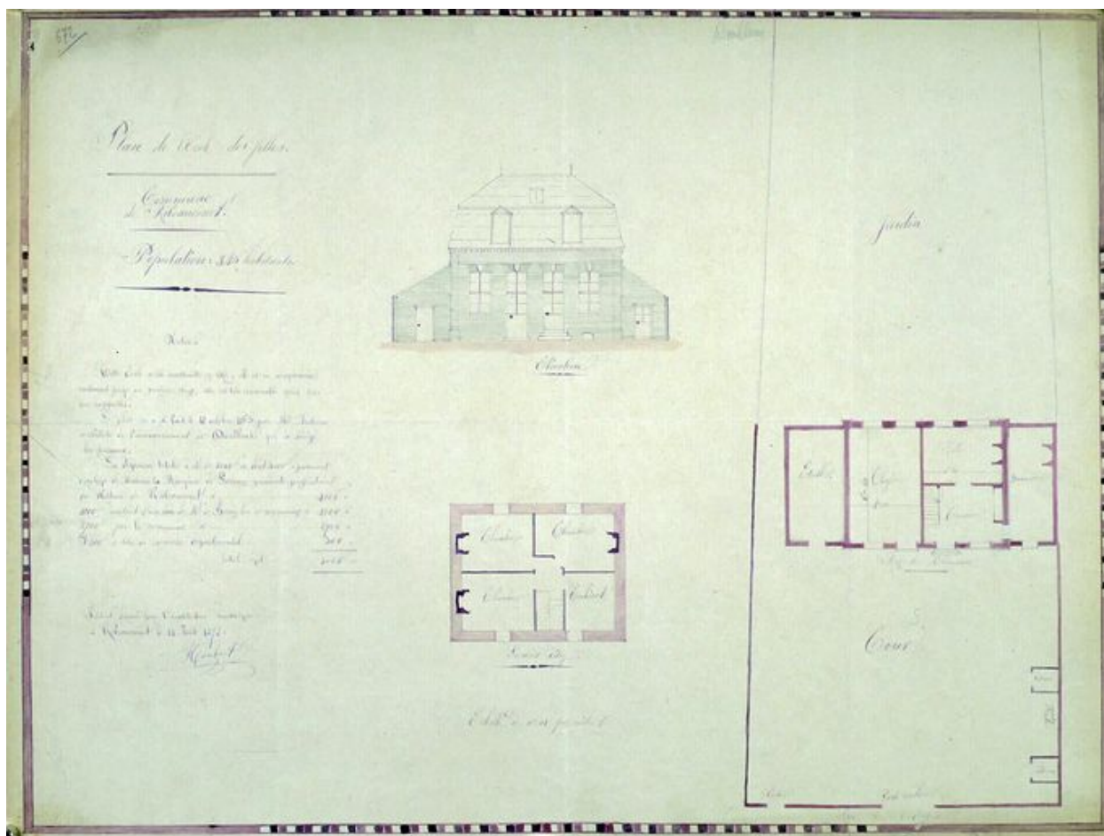
Plan et élévation par A. Houtier, 1878 (AD Somme ; 99 T 3807/672).
