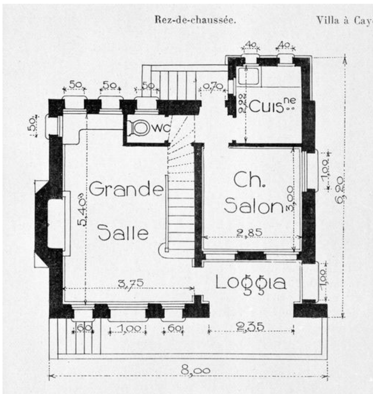
Plan du rez-de-chaussée (AD Somme ; 1 J 3584/11).
