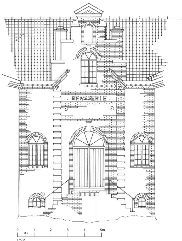
59 HOUPLINES Brasserie ROUSSEL DELOBEL Elévation sur cour Dessin Eddy Stein. 1990 Inventaire général Nord-Pas de Calais
