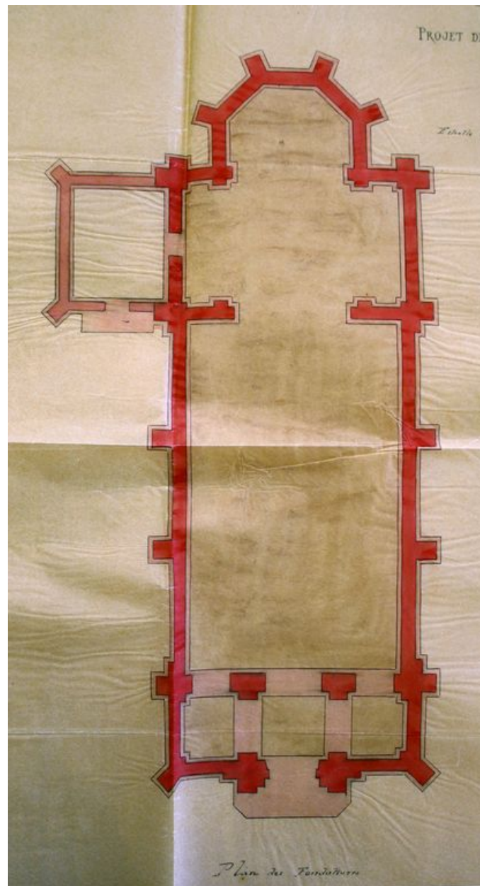
Plan des fondations de la nouvelle église, par Herbault (architecte), 25 avril 1866 (AD Somme ; 99 O 3775).
