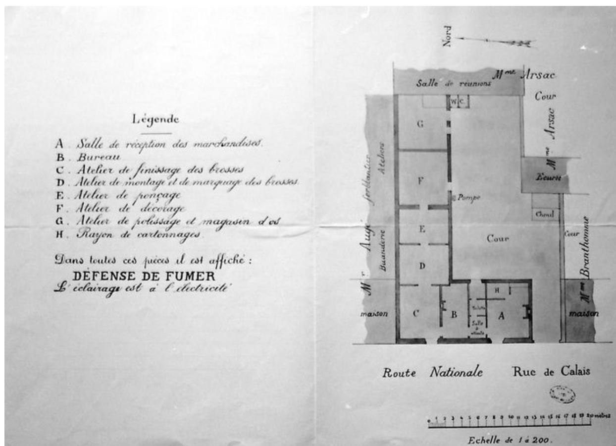
Plan détaillé de la broserie en 1929 (AD Oise, Mp 2518).
