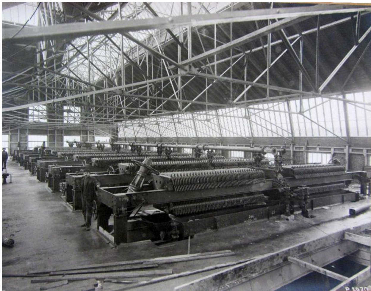
Atelier des filtres presses, 6 novembre 1922 (AD Somme ; 49 Fi 22).
